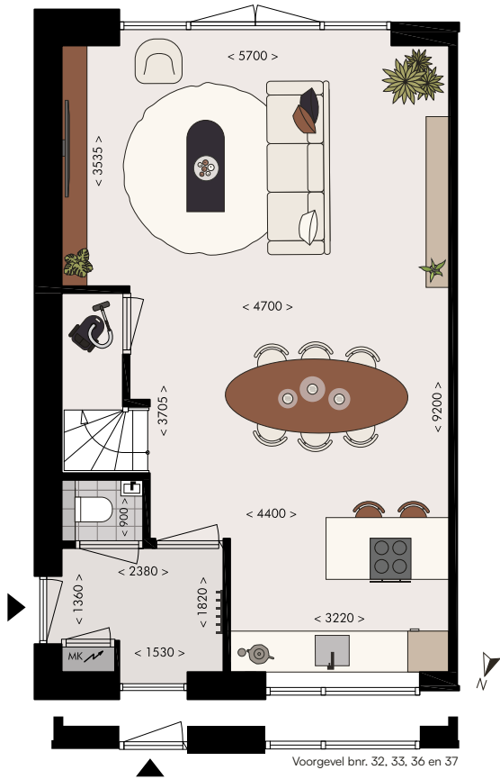
Winterkoning Bnr. 32, 34, 36 en 38 | Bnr. 31, 33, 35 en 37 gespiegeld Begane grond
