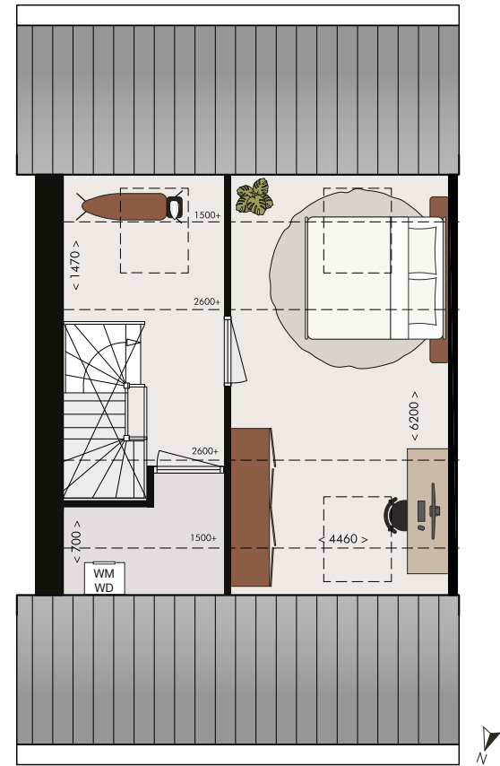
Winterkoning Bnr. 32, 34, 36 en 38 | Bnr. 31, 33, 35 en 37 gespiegeld Tweede verdieping
