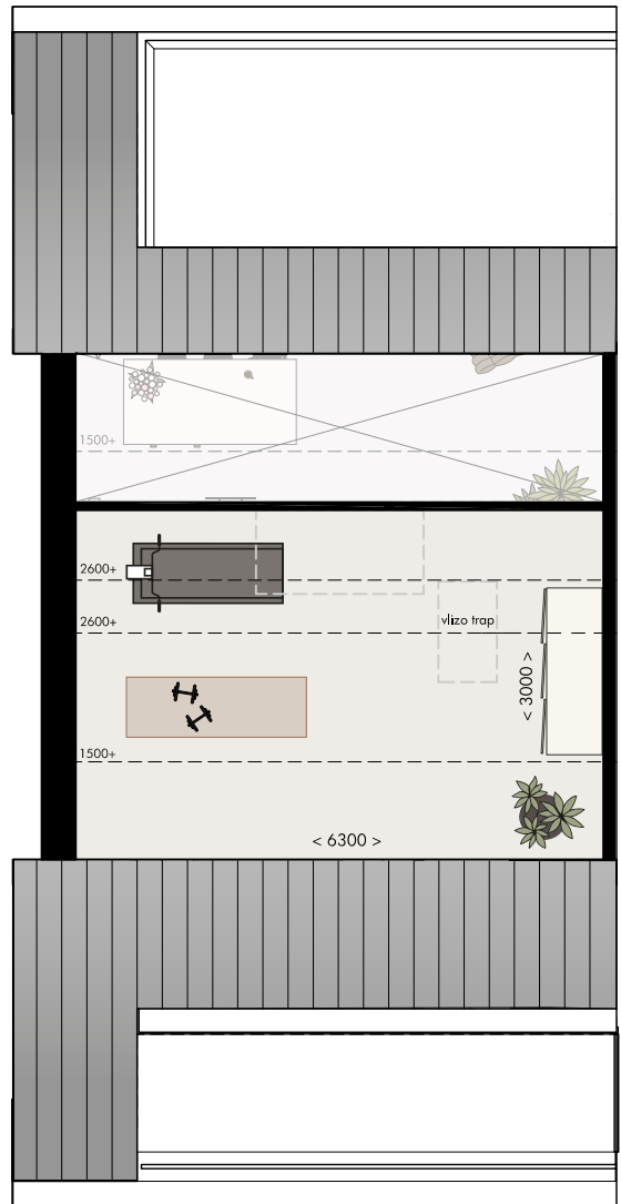
IJsvogel Bnr. 44 | Bnr. 46 gespiegeld Tweede verdieping
