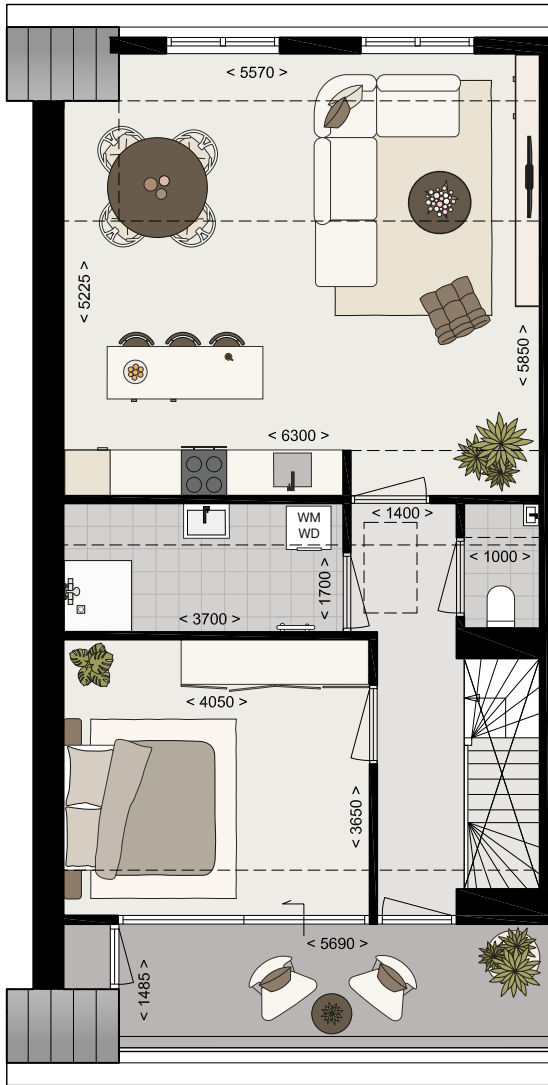
IJsvogel Bnr. 44 | Bnr. 46 gespiegeld Eerste verdieping
